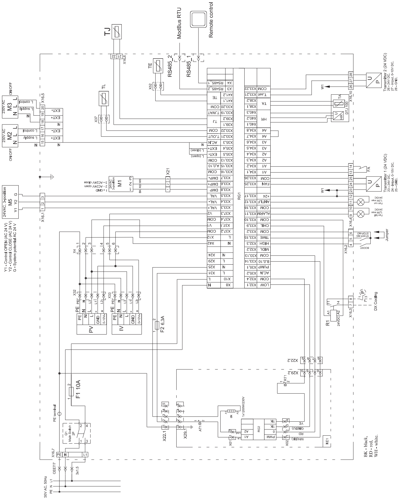
Рис. 18.2. Схема электрических подключений LV-PACU 700 VE-V4-ECO
