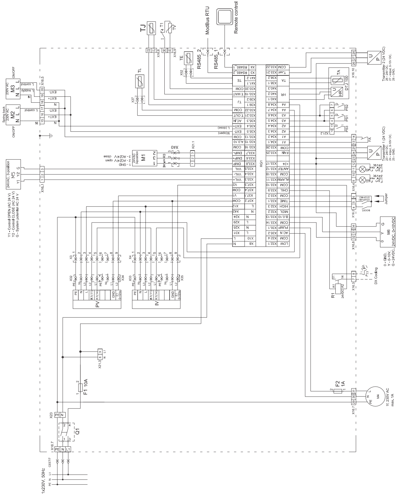
Рис. 18.7. Схема электрических подключений LV-PACU 1900 VW-V4-ECO
