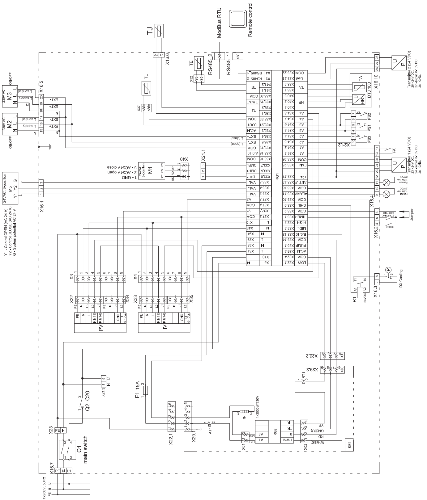
Рис. 18.6. Схема электрических подключений LV-PACU 1900 VE-V4-ECO
