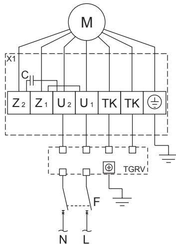
Схема подключения № 1 (см. «Технические характеристики»)
