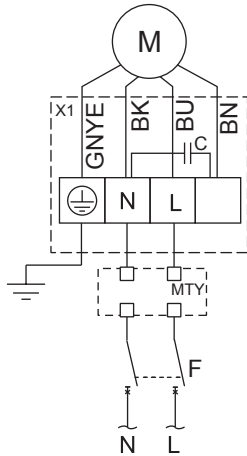
Схема подключения № 3 (см. «Технические характеристики»)
