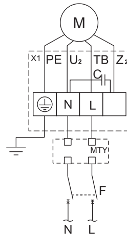
Рис. 2. Схемы электрических подключений.
