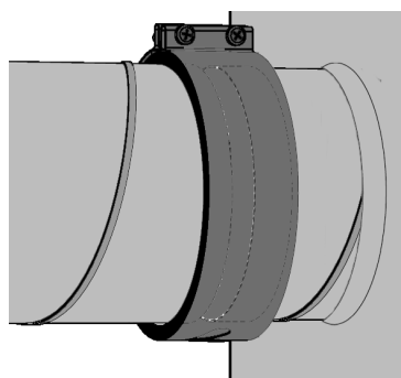
Рис. 7.2. Пример использования быстросъемного хомута LV-MDC
