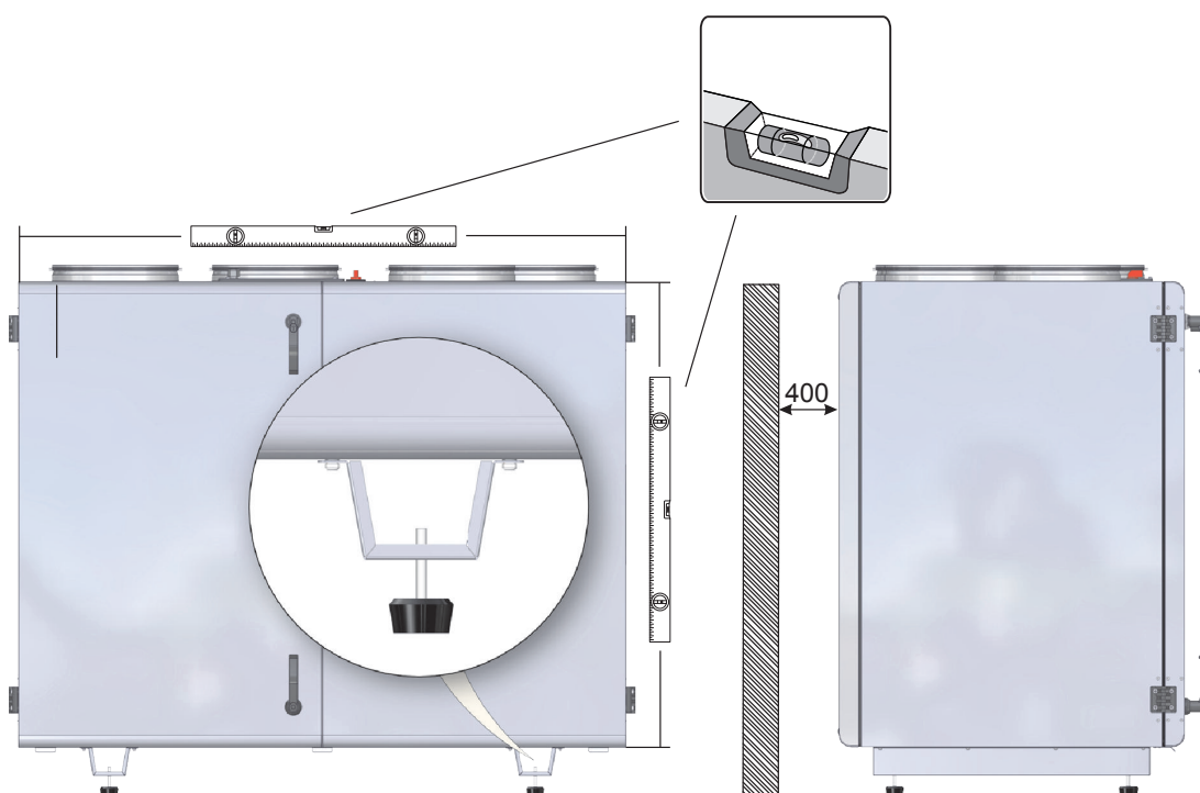
Рис. 7.1. Монтаж вентустановки
