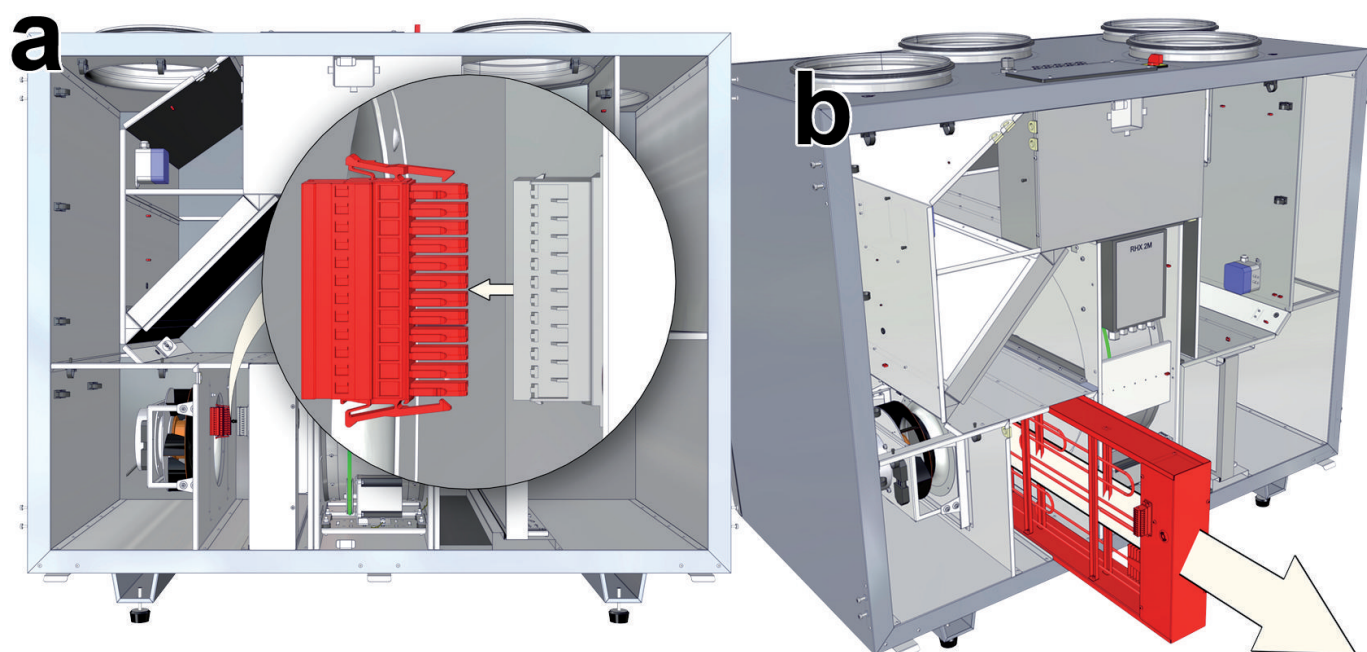
Рис. 13.5. Демонтаж электронагревателя LV-RACU 1200–1900 VE-V4-ECO. а) открыть сервисную дверцу и разъединить контактную группу; б) вытащить электронагреватель
