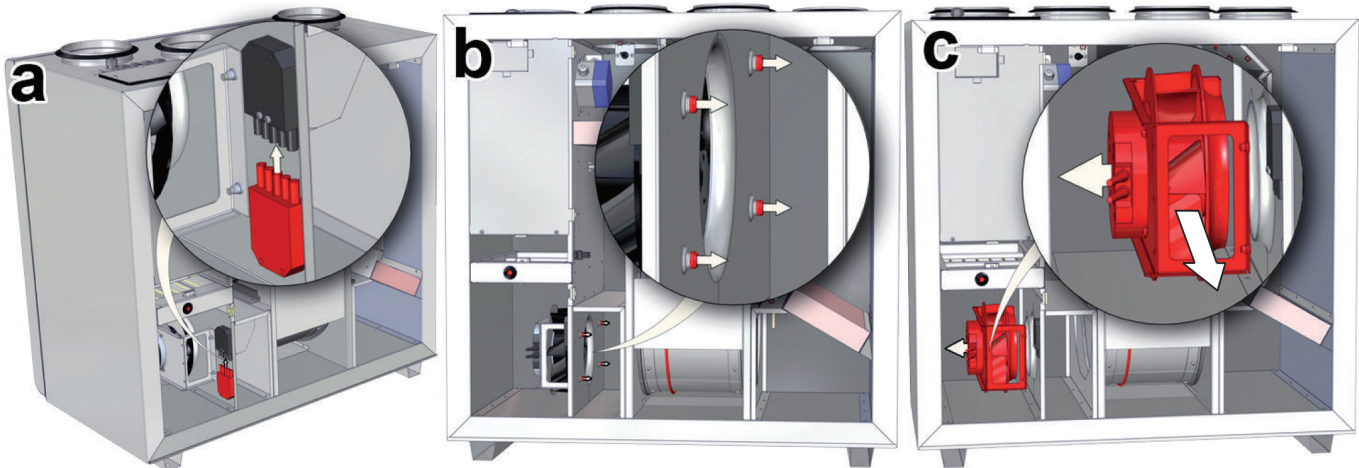
Рис. 13.1. Демонтаж вентилятора LV-RACU 400 V-V4-ECO.
