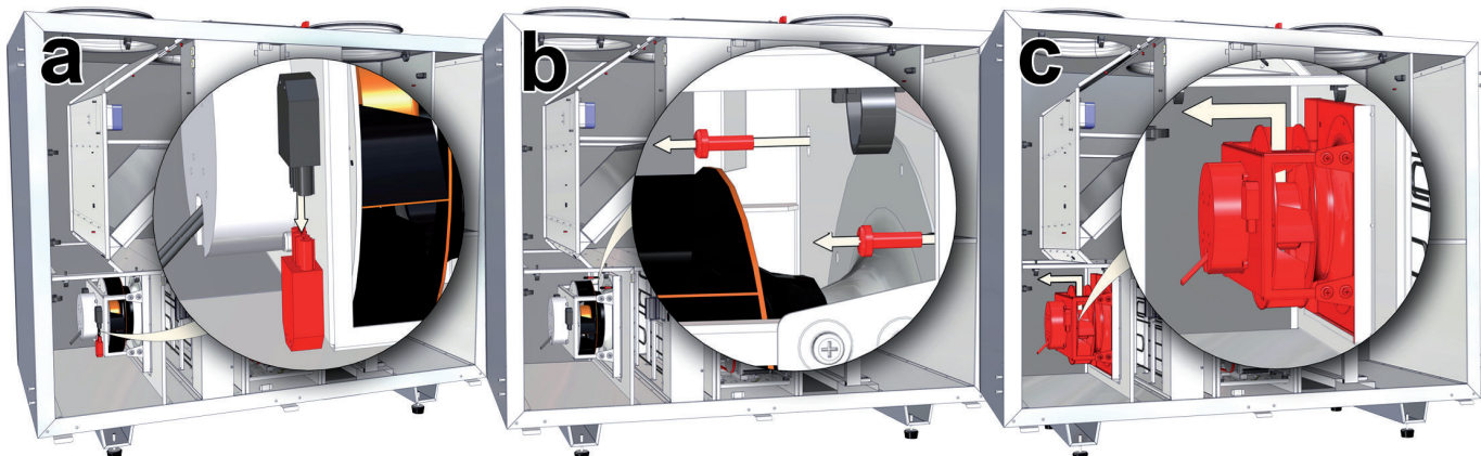
Рис. 13.3. Демонтаж вентилятора LV-RACU 1200–1900 V-V4-ECO.
