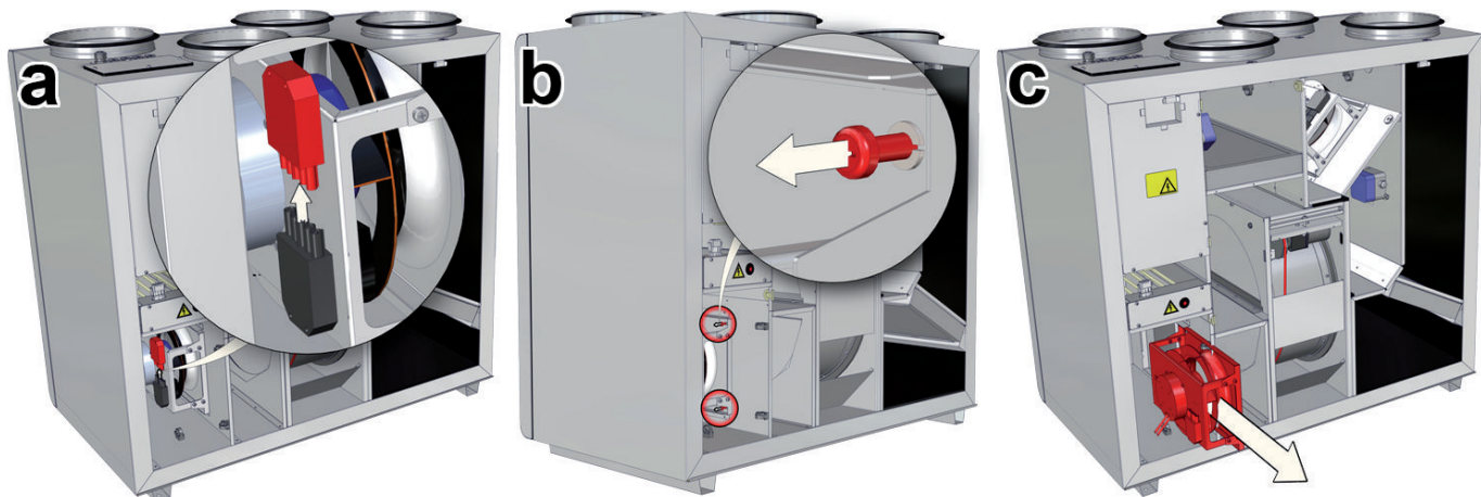
Рис. 13.2. Демонтаж вентилятора LV-RACU 700 V-V4-ECO.
