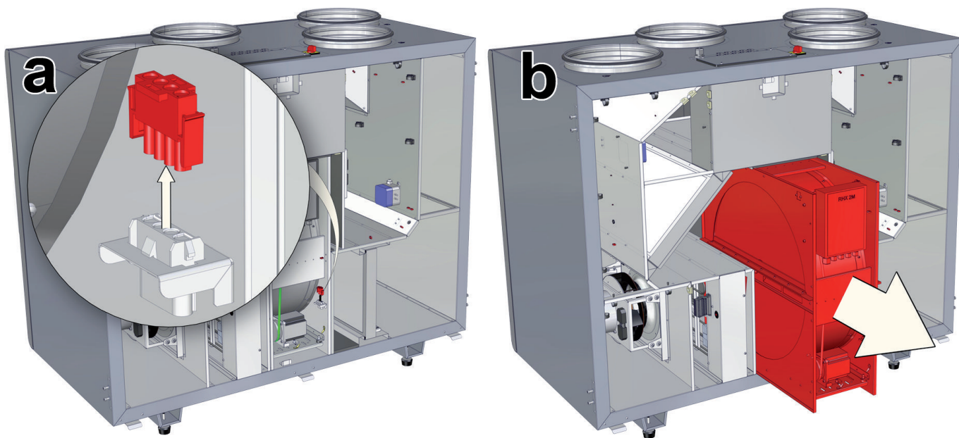
Рис. 13.7. Демонтаж регенератора LV-RACU 1200–1900 V-V4-ECO. а) открыть сервисную дверцу и разъединить контактную группу; б) вытащить регенератор
