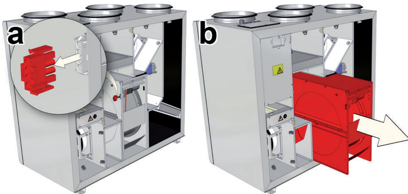
Рис. 13.6. Демонтаж регенератора LV-RACU 400–700 V-V4-ECO. а) открыть сервисную дверцу и разъединить контактную группу; б) вытащить регенератор
