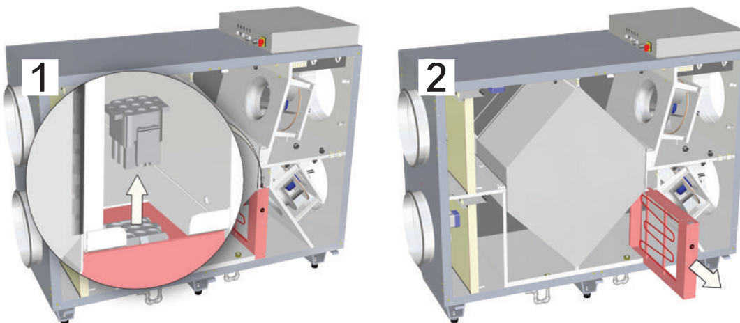
Рис. 15.3. Демонтаж электрического нагревателя LV-PACU 1900HE-V4-ECO. 1) открыть сервисную дверцу и разъединить контактную группу; 2) вытащить электронагреватель
