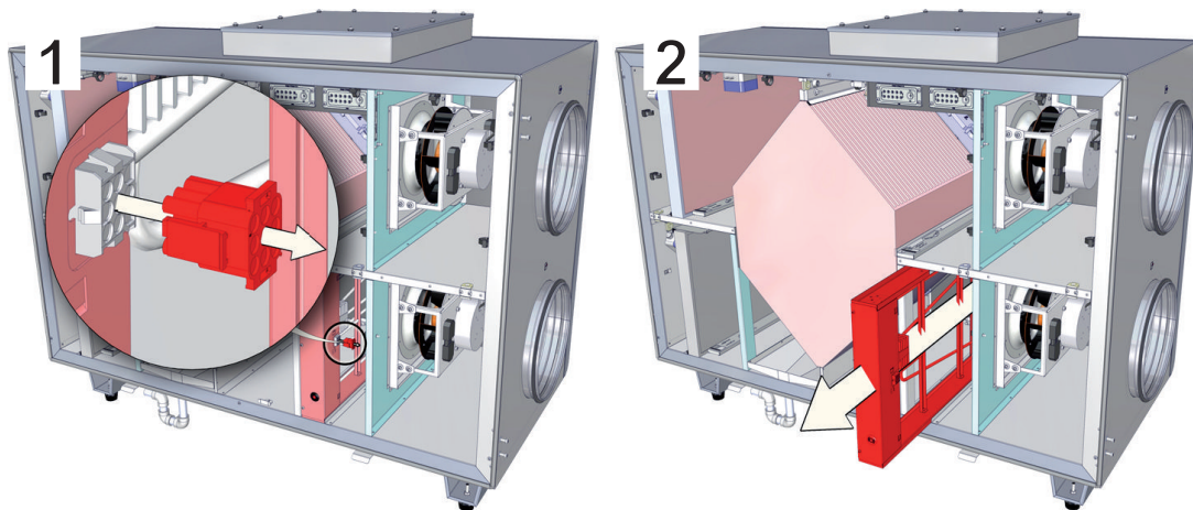
Рис. 15.2. Демонтаж электрического нагревателя LV-PACU 1200HE-V4-ECO. 1) открыть сервисную дверцу и разъединить контактную группу; 2) вытащить электронагреватель
