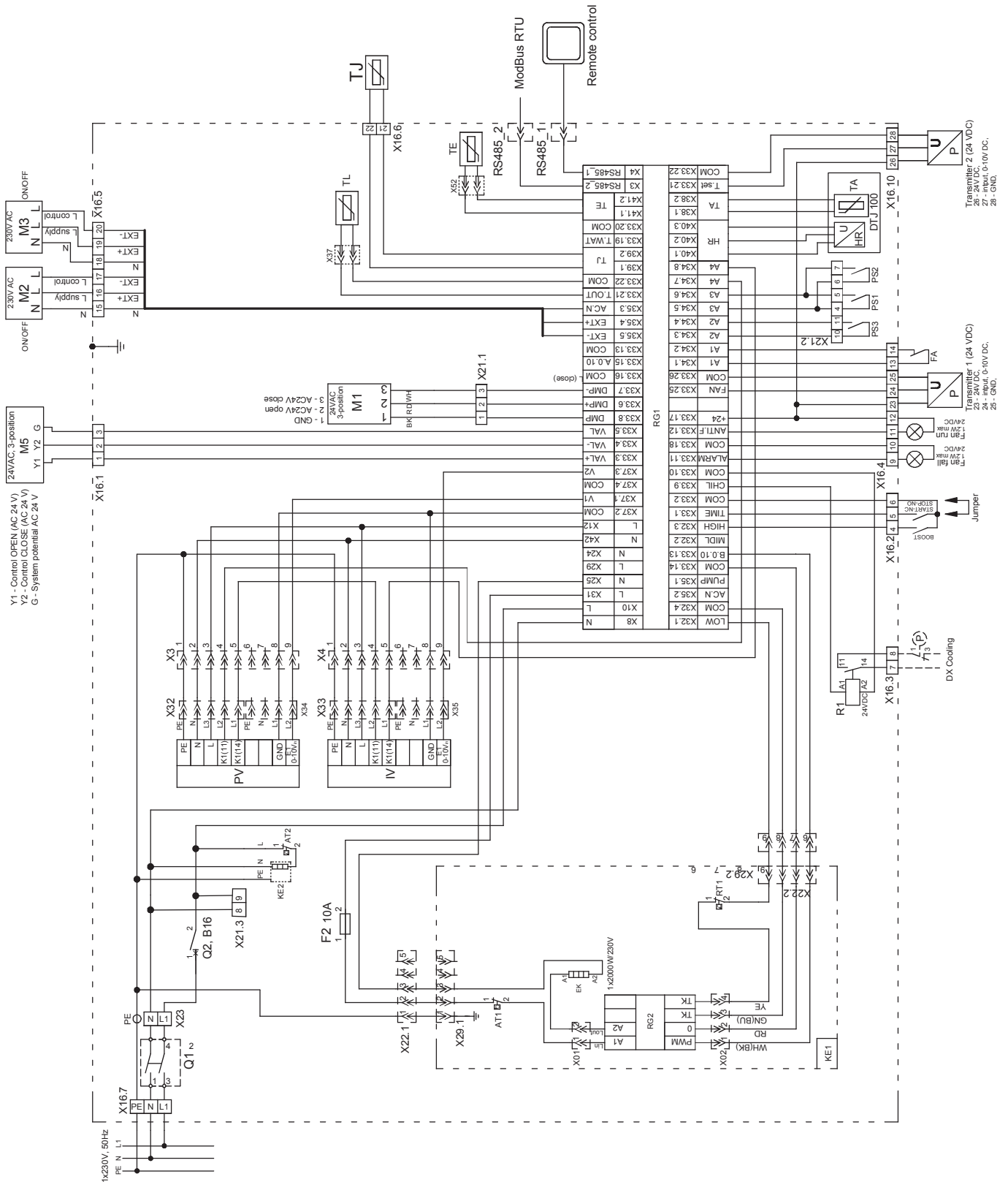
Рис. 18.4. Схема электрических подключений LV-PACU 1200, 1900 HE-V4-ECO
