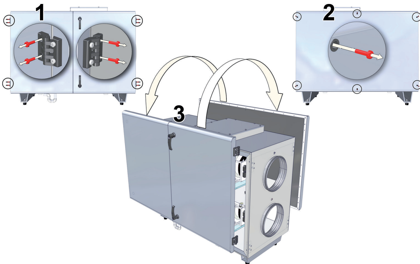
Рис. 8.2. Изменение стороны обслуживания LV-PACU 1200 H-V4-ECO.
