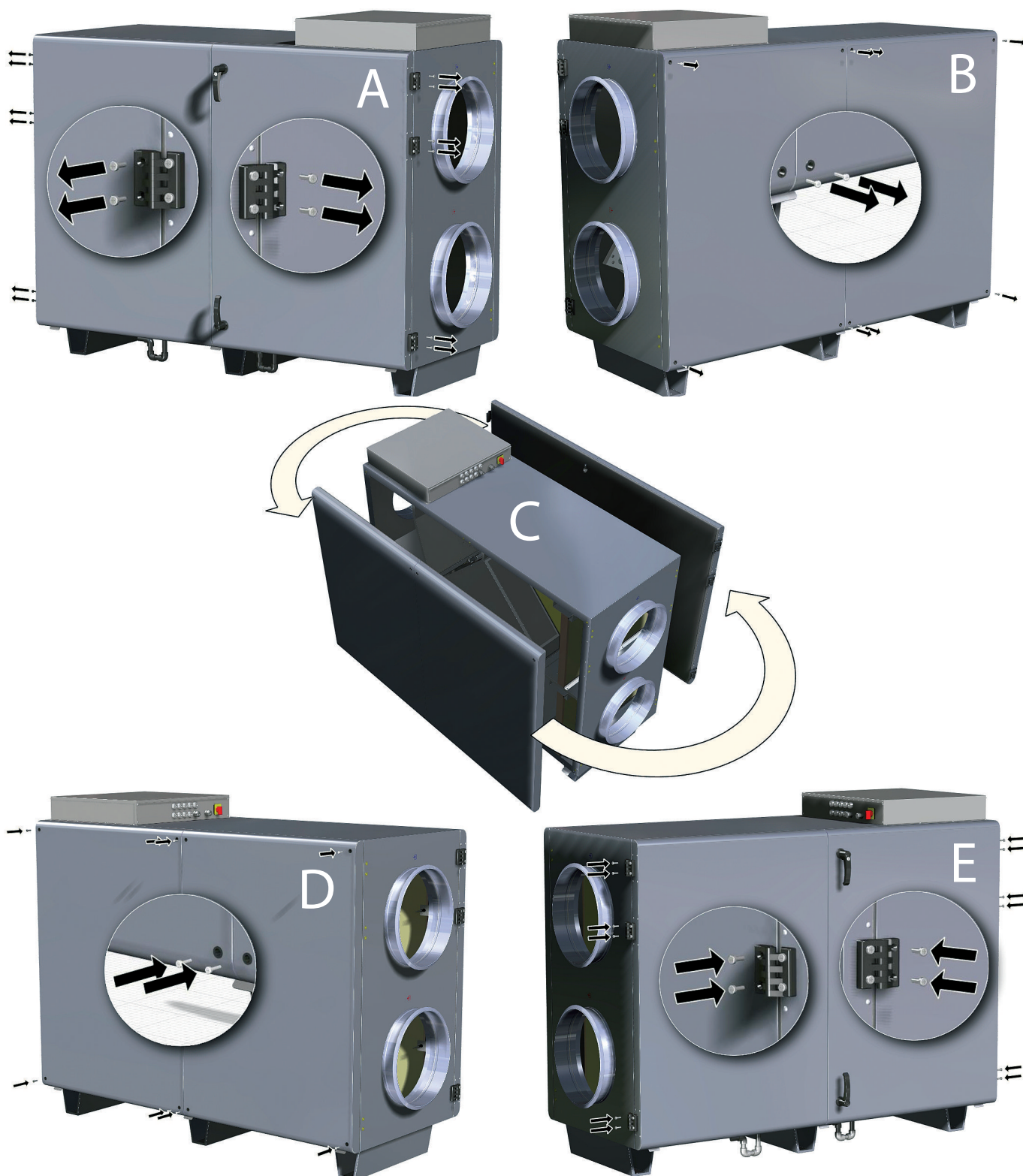
Рис. 8.3. Изменение стороны обслуживания LV-PACU 1900 H-V4-ECO.
