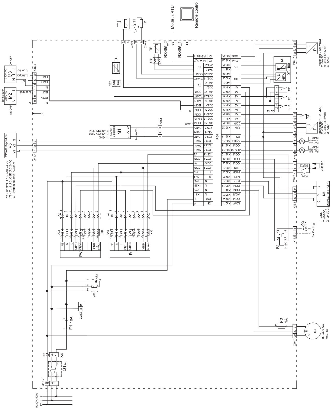
Рис. 18.5. Схема электрических подключений LV-PACU 1200 HW-V4-ECO
