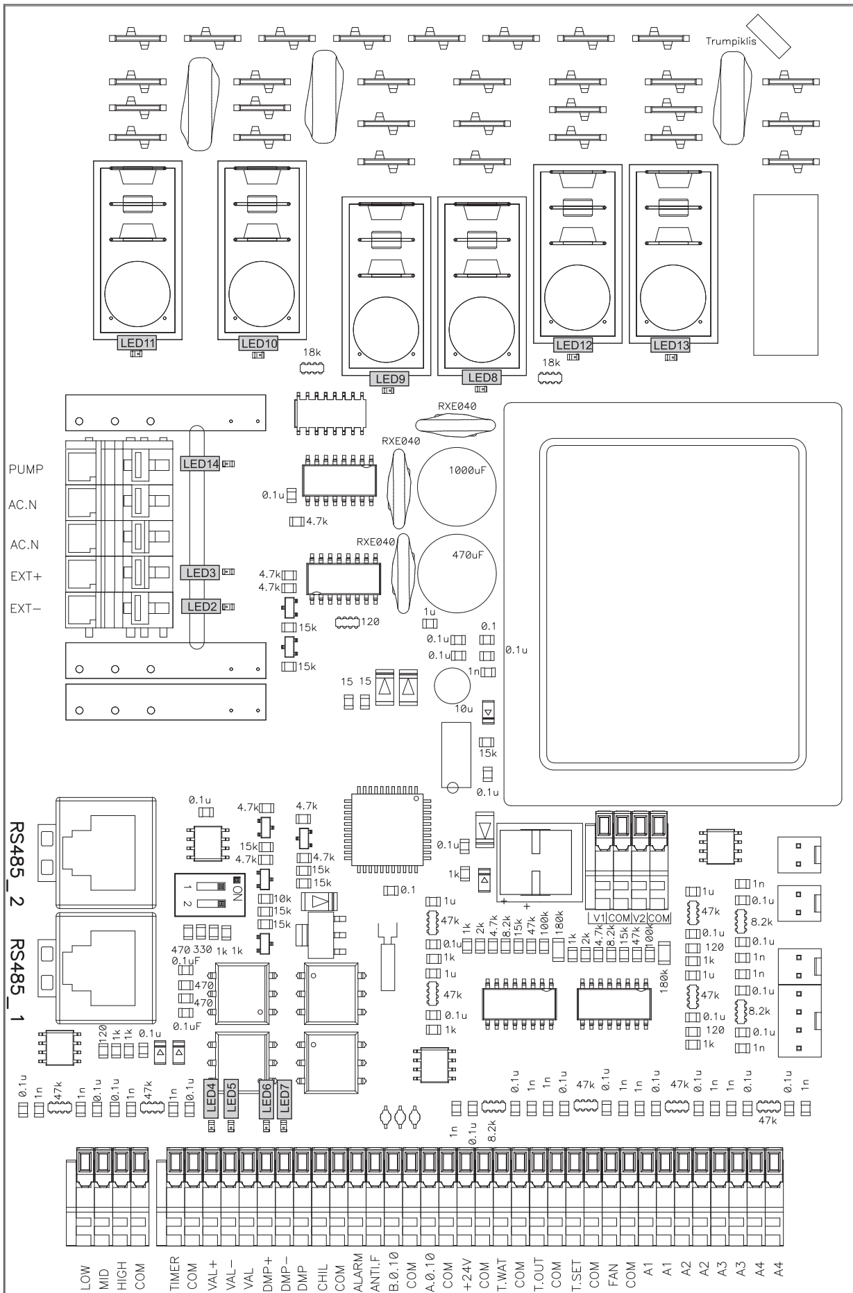
Рис. 18.1. Плата автоматики RG1
