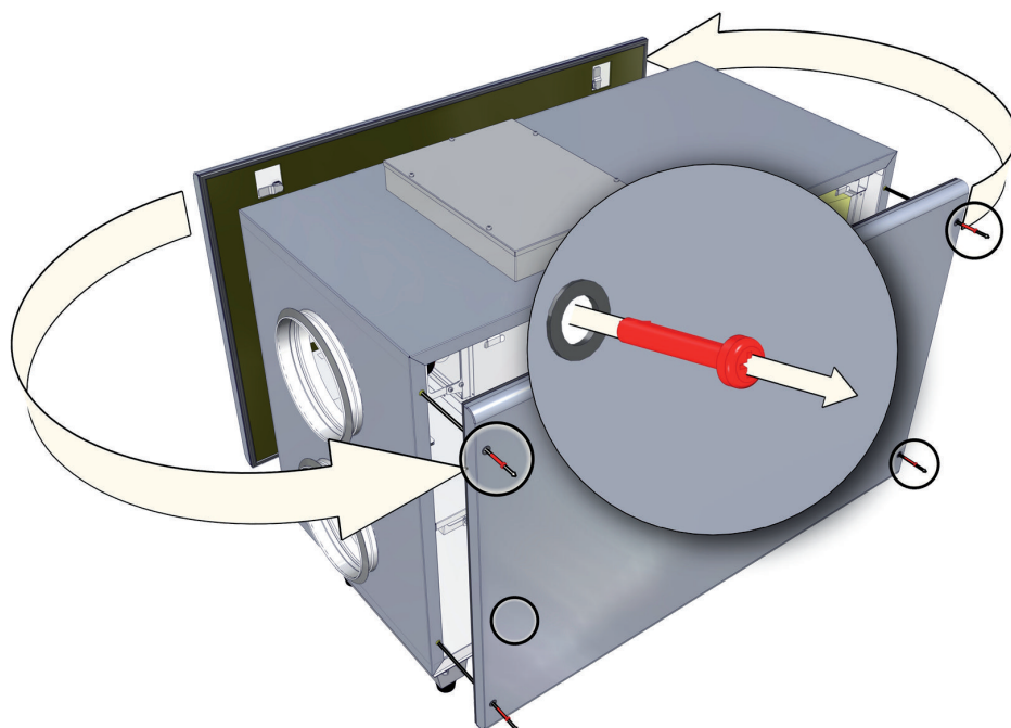
Рис. 8.1. Изменение стороны обслуживания LV-PACU 700 H-V4-ECO.
