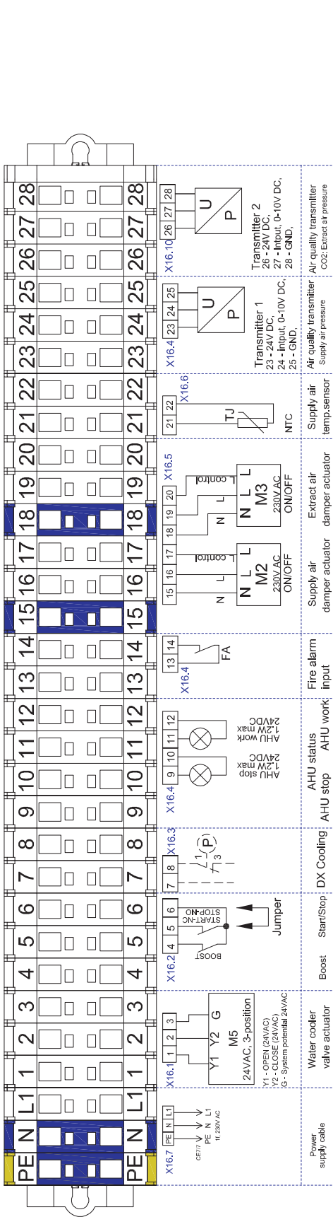
Рис. 18.7. Клеммная колодка X16 для комплектов с электрическим нагревателем
