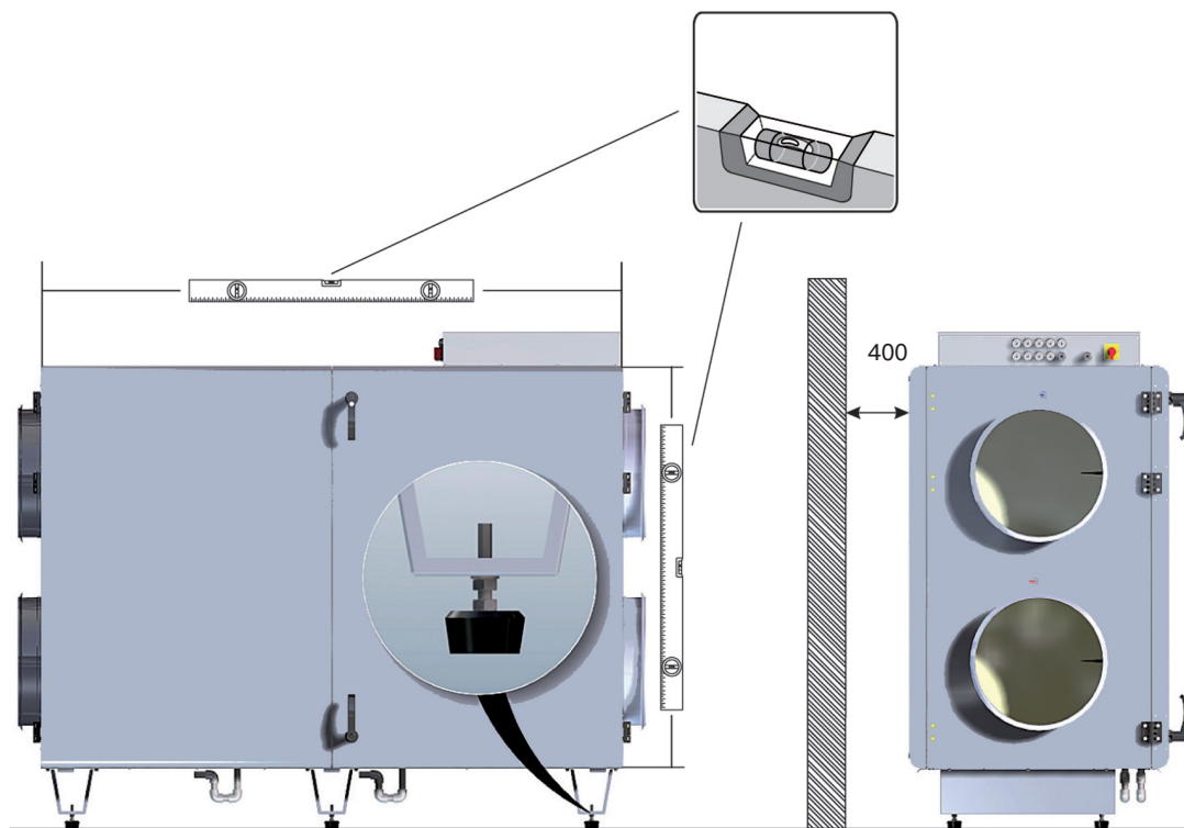
Рис. 7.1. Монтаж вентустановки
