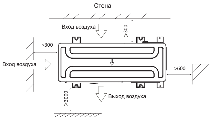
Монтаж нескольких наружных блоков в ограниченном пространстве
