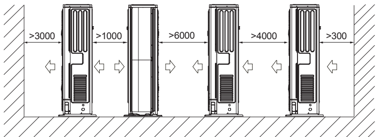
Монтаж нескольких наружных блоков в ограниченном пространстве
