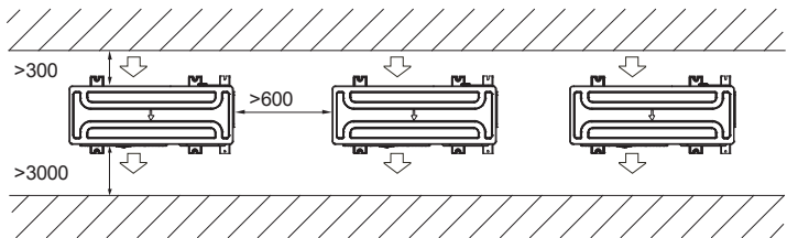
Монтаж нескольких наружных блоков в ограниченном пространстве
