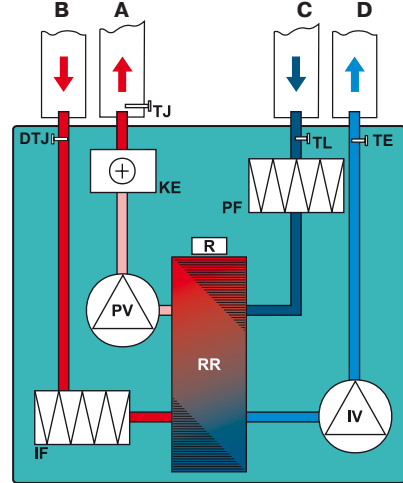
LV-RACU 400 VER-V4
