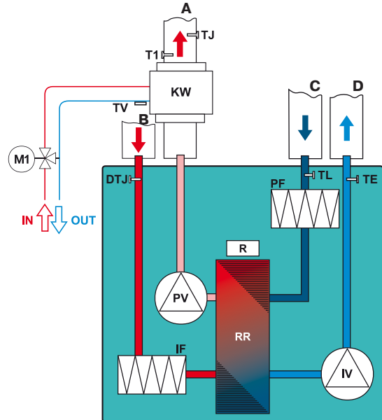
LV-RACU 400 VWR-V4
