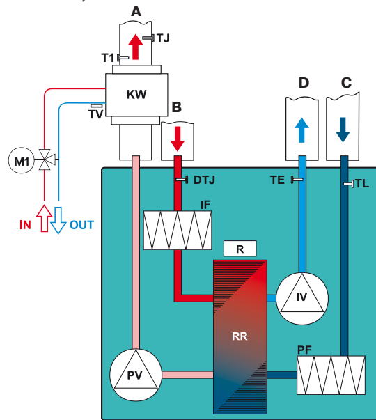
LV-RACU 700, 1200 VWR-V4
