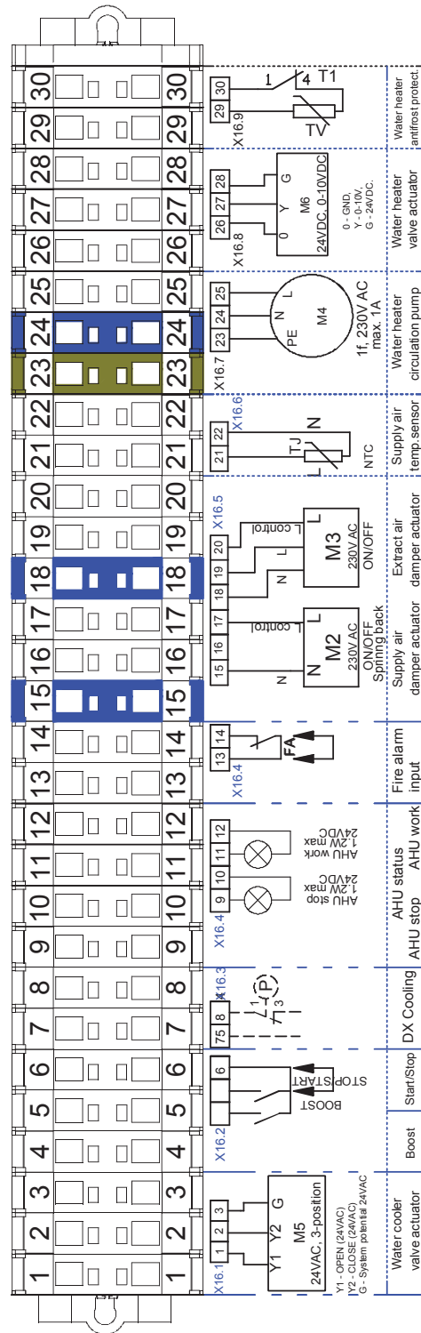
Рис. 14.7. Клеммная колодка X16 для Укомплектов с водяным нагревателем
