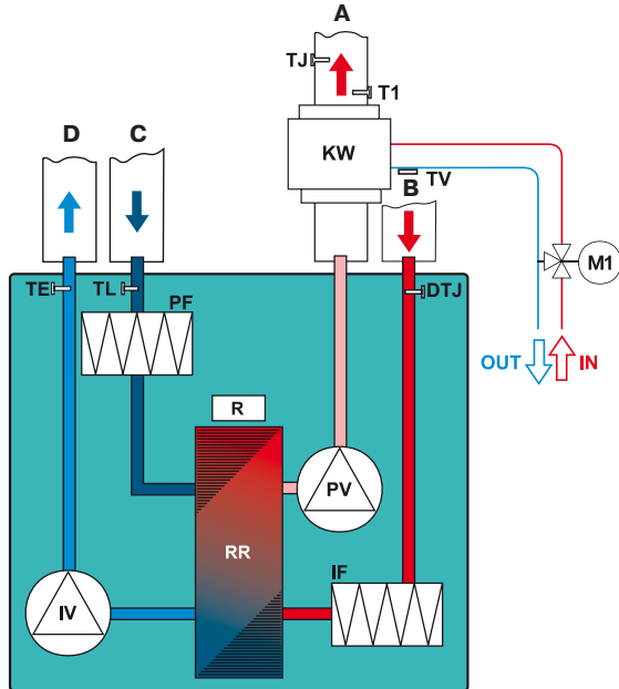
LV-RACU 400 VWL-V4
