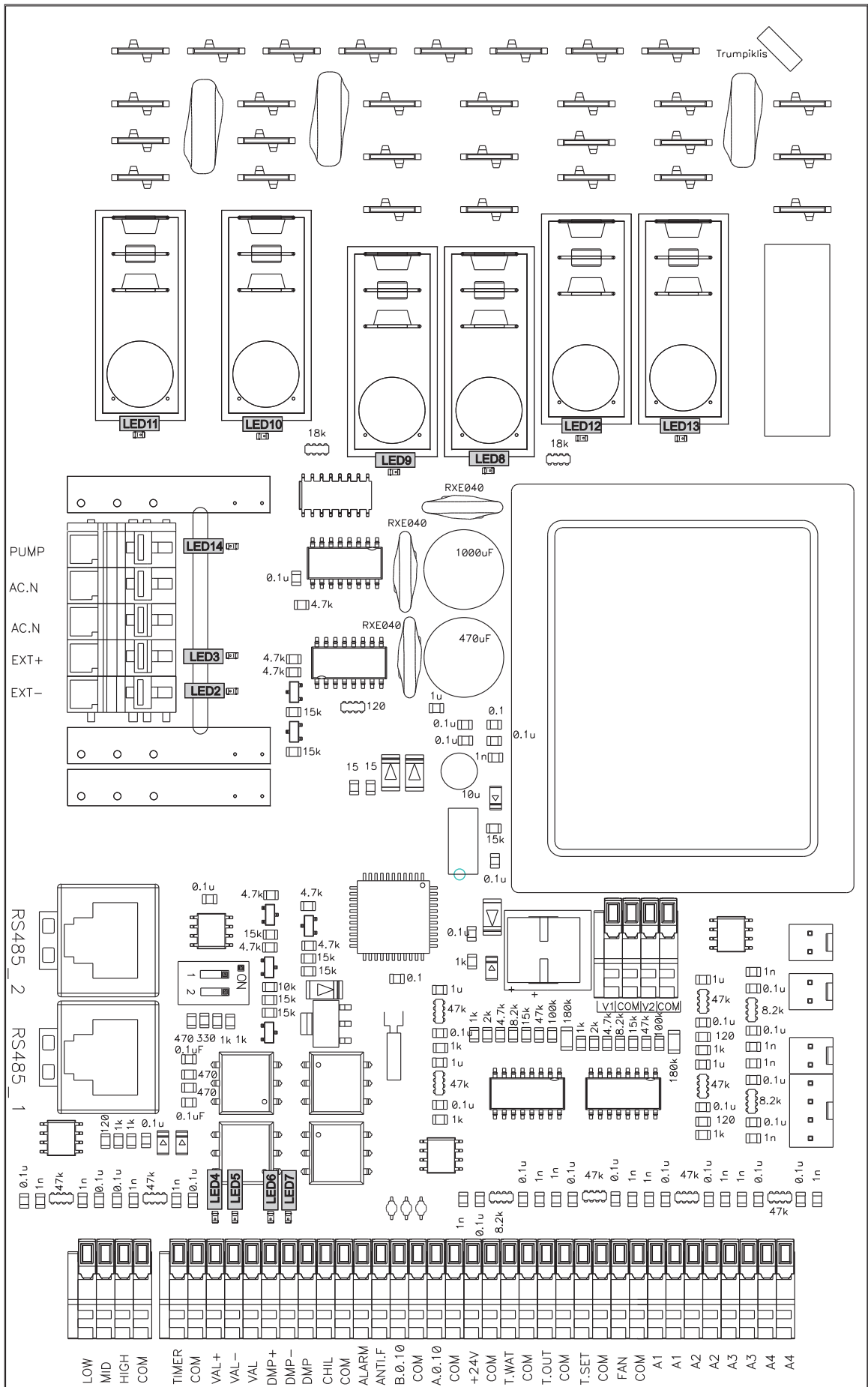
Рис. 14.1. Плата автоматики RG1
