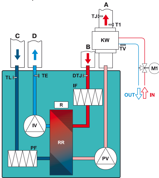
LV-RACU 700, 1200 VWL-V4
