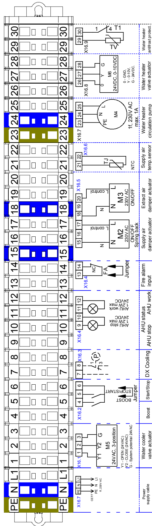
Рис. 12.9. Клеммная колодка X16 для комплектов с водяным нагревателем
