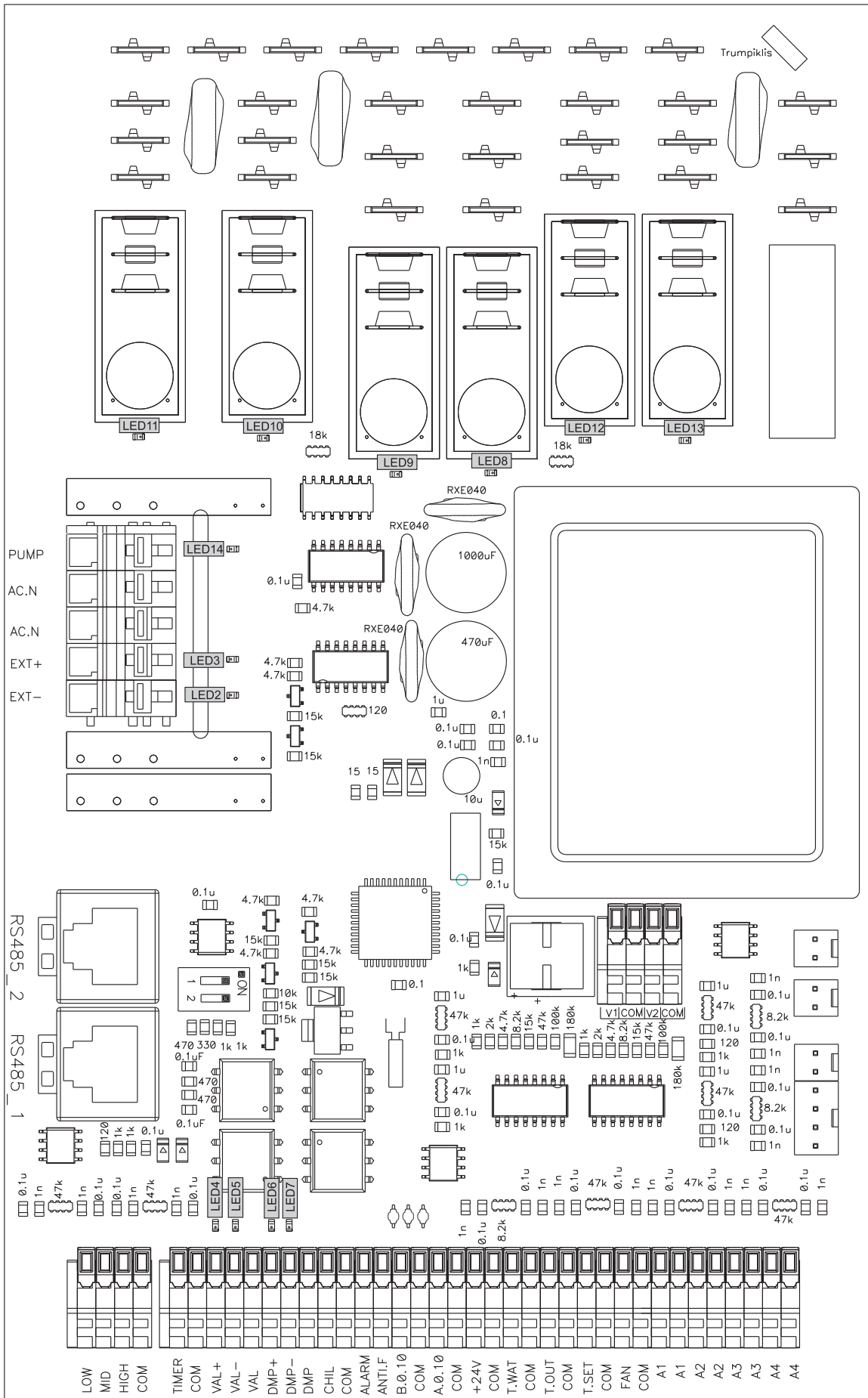
Рис. 12.1. Плата автоматики RG1
