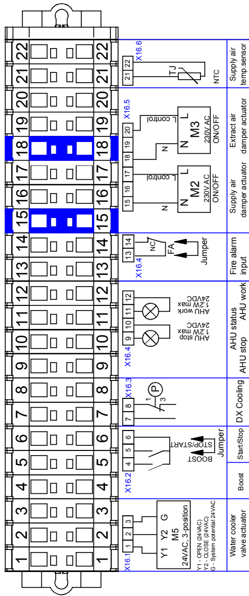
Рис. 12.8. Клеммная колодка X16 для комплектов с электрическим нагревателем
