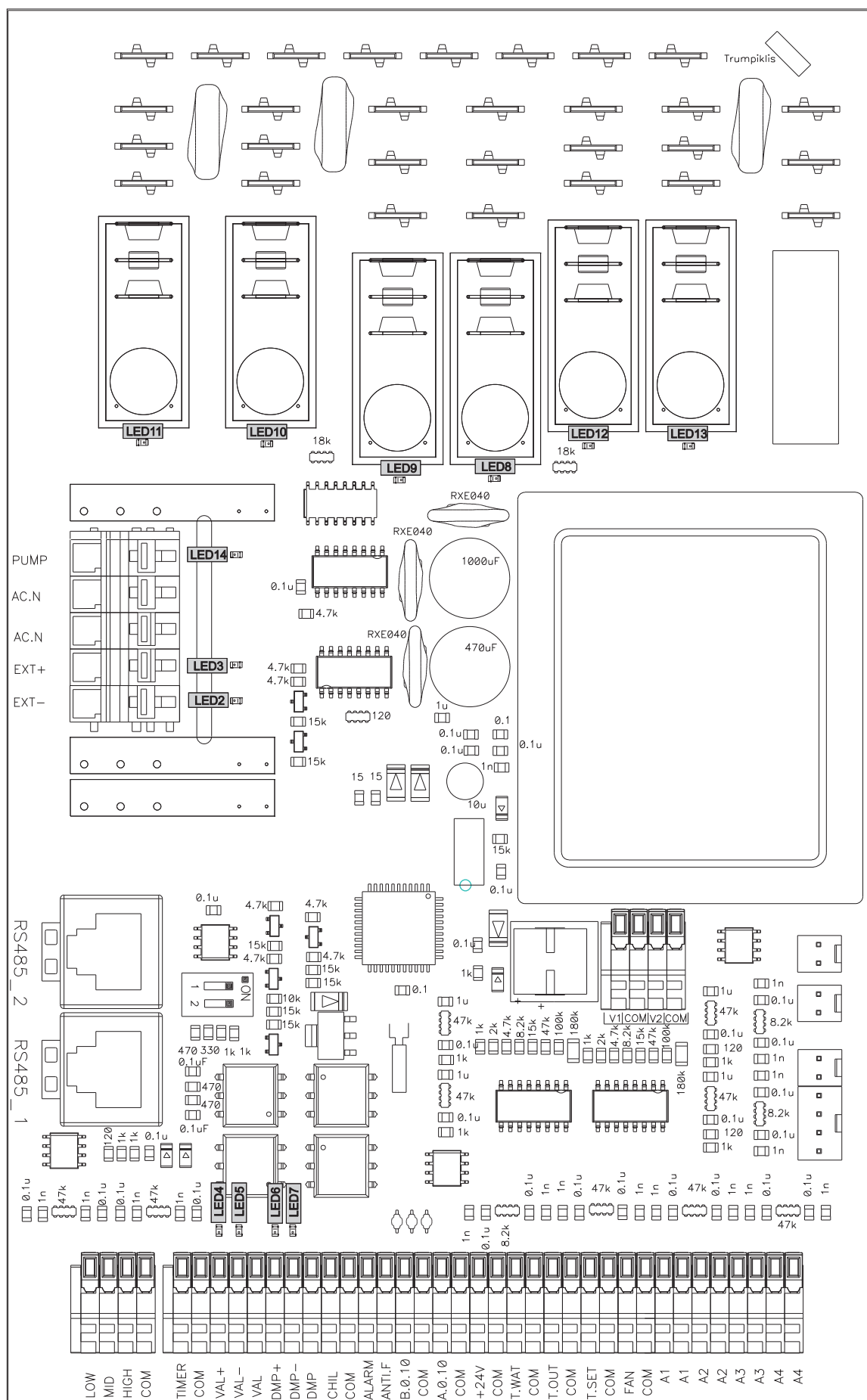
Рис. 16.1. Плата автоматики RG1
