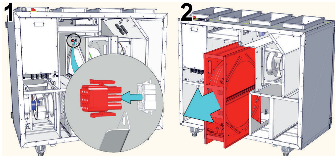
Рис. 13.2. Демонтаж регенератора LV-RACU 2500–5500 V-V4-ECO.
