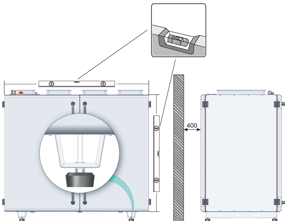
Рис. 7.1. Монтаж вентустановки
