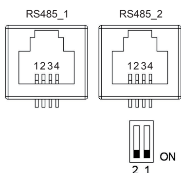
Рис. 12.1. Разъемы RS485 и микропереключатели сопротивления.
