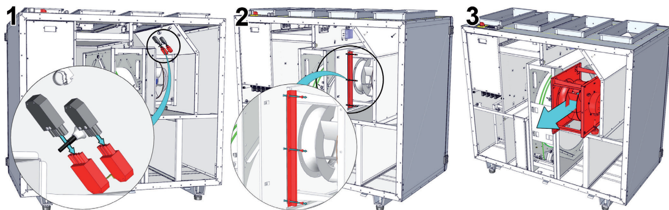
Рис. 13.1. Демонтаж вентилятора LV-RACU 2500–5500 V-V4-ECO.
