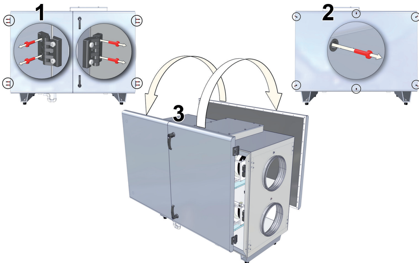
Рис. 7.2. Изменение стороны обслуживания LV-PACU 1000, 1500, 1900 H-V4.
