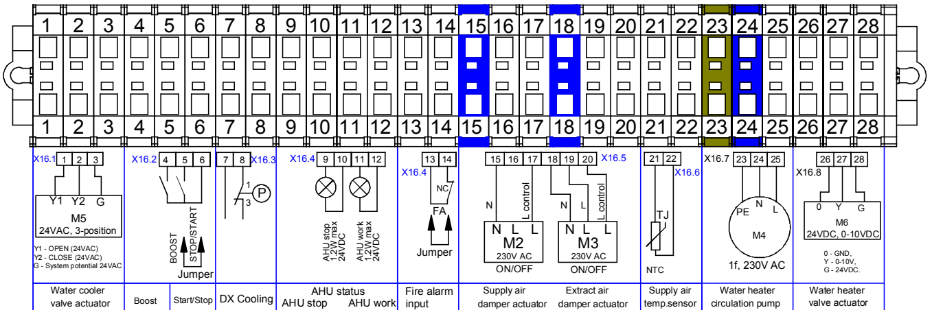
Рис. 16.11. Клеммная колодка X16 для для компактов с водяным нагревателем
