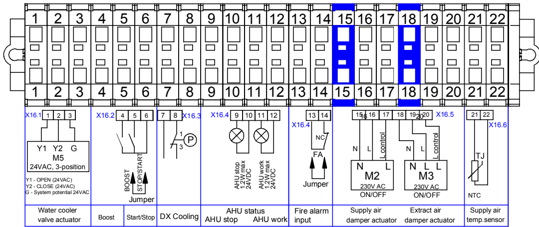
Рис. 16.10. Клеммная колодка X16 для компактов с электрическим нагревателем
